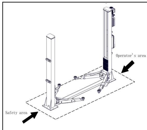
Abb. 8 Arbeitsbereich
