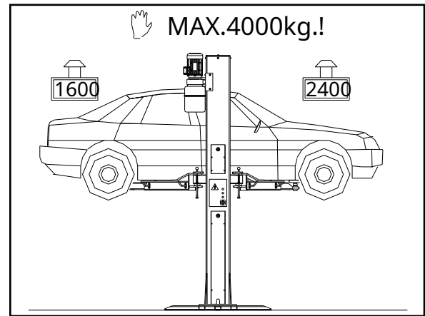
Abb. 7 Gewichtsverteilung
