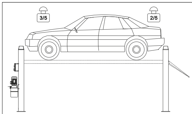
Rys. 12 Rozkład masy
